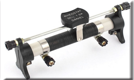
Rheostat
